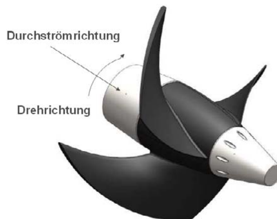
Abb. 13: Pentair Nijhuis Turbine (GRÜNIG, 2013)
